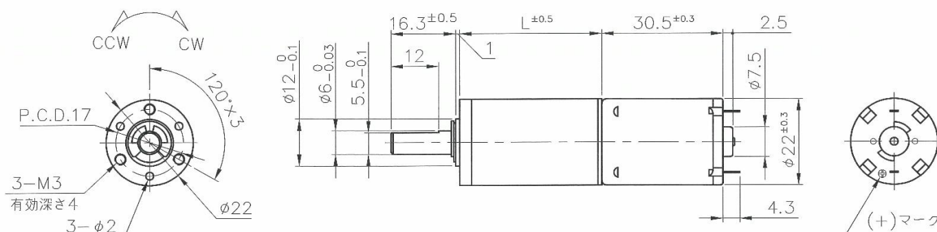
【外径図】
