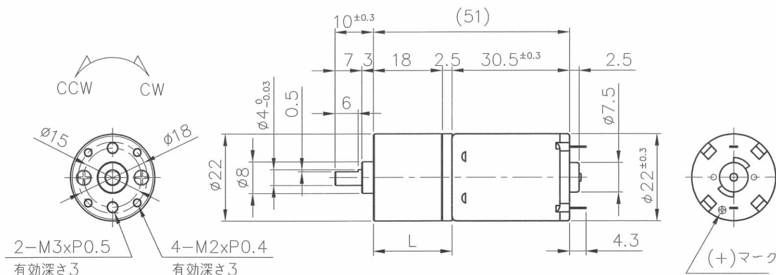
【外径図】
